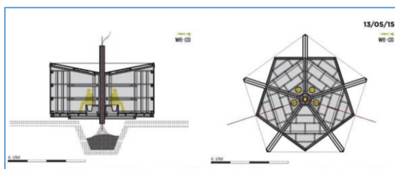
Dessin de travail des latrines mobiles multi-cabines
